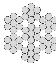
6x7+IWS.A2
