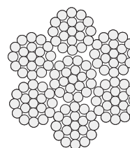
6x19+IWS.A2
